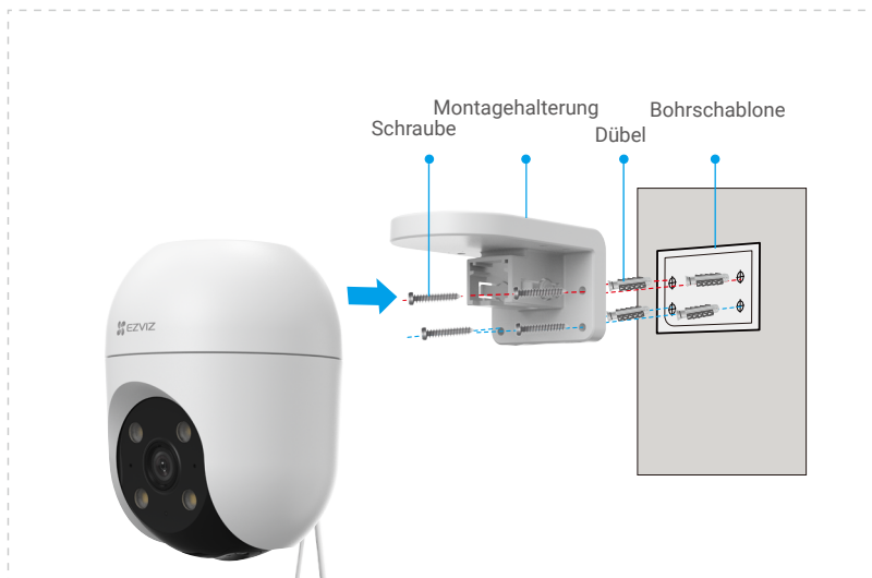
Abb. 2 Wandmontage
