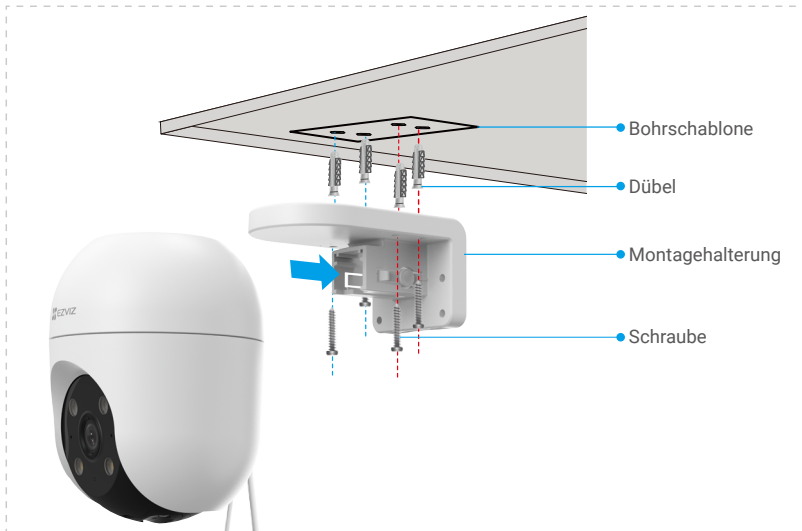
Abb. 1 Deckenmontage
